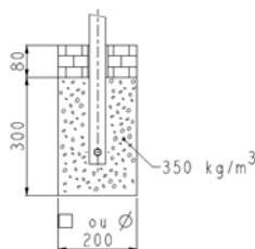
Scellement direct
